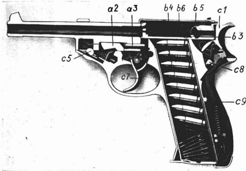
Pistole 38, aufgeschnitten
